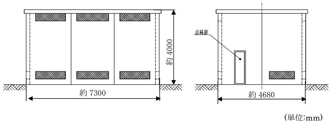
図 3.6.4-1 コンクリートモジュール概略図
